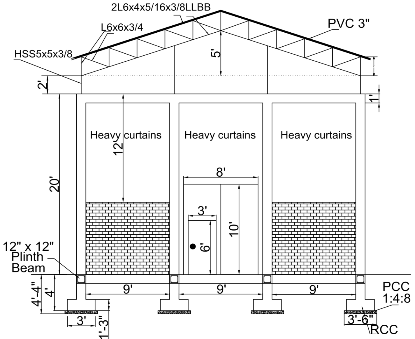
ELEVATION 1:2:4
